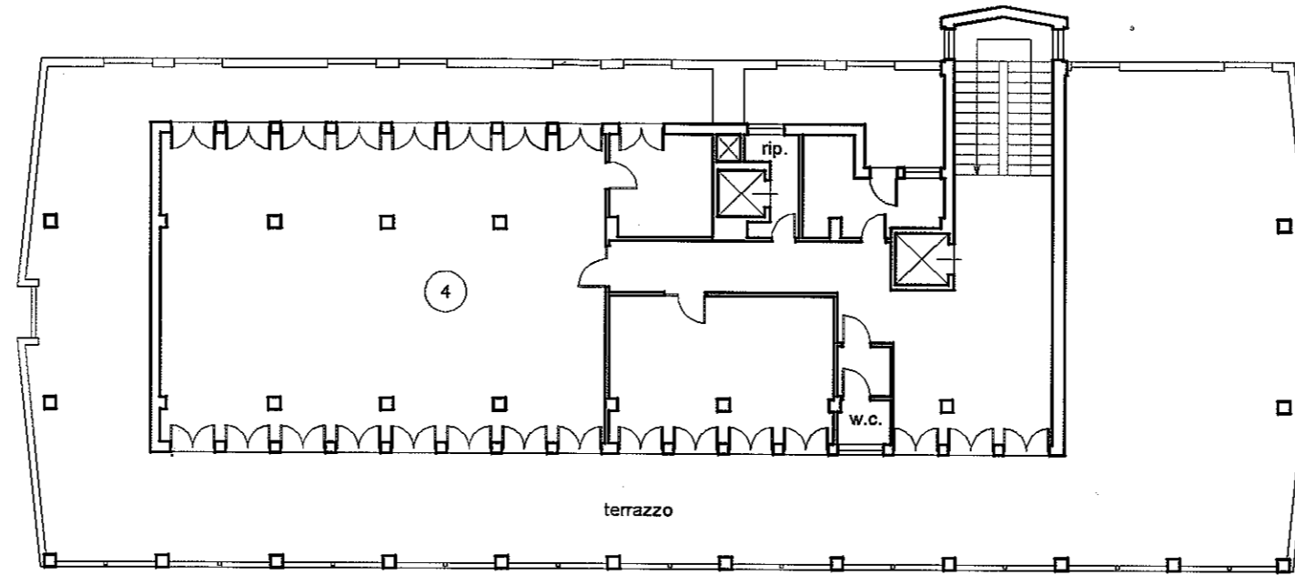
H= 3,00 mt. Piano terzo
